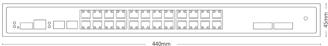
Вид спереди
